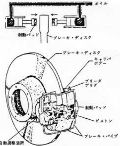
ディスクブレーキ装置
